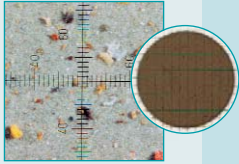
取自CJC™精滤器安装前的油样
