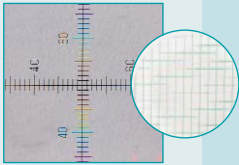
取自CJC™精滤器安装后的油样
